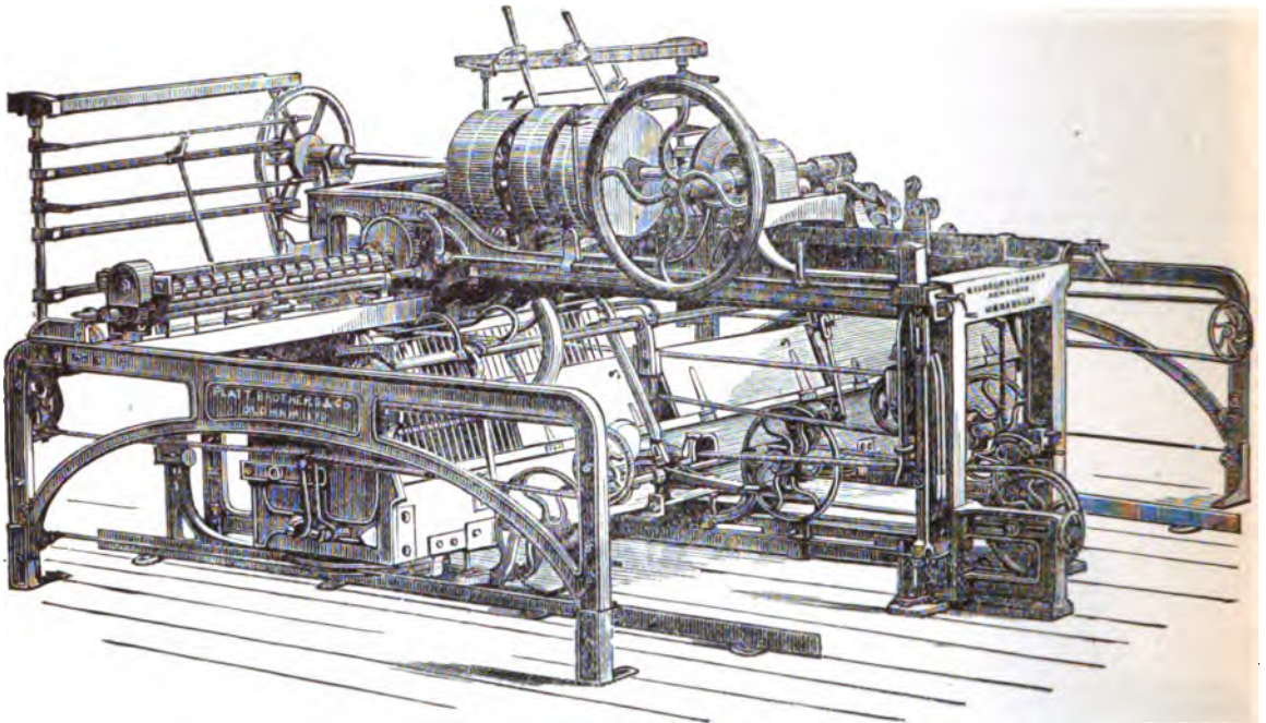
FIG. 13.—Hand-Mule.
