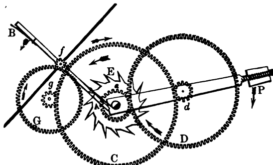
FIG. 20.—Gravity Train Remontoire.
