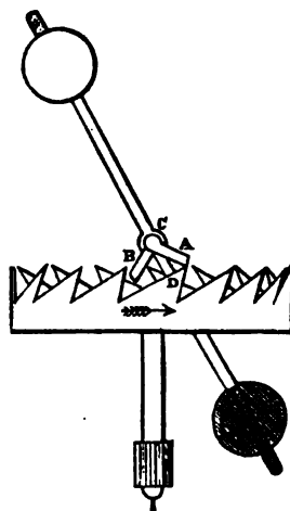
Fig. 3.—Recoil Escapement.
