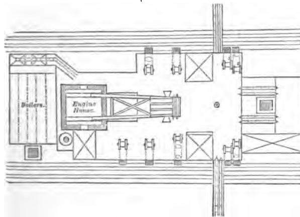
FIG. 23.—Plan.
