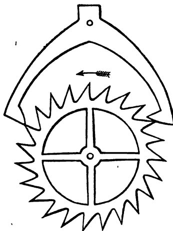
Fig. 4.—Anchor Escapement.
