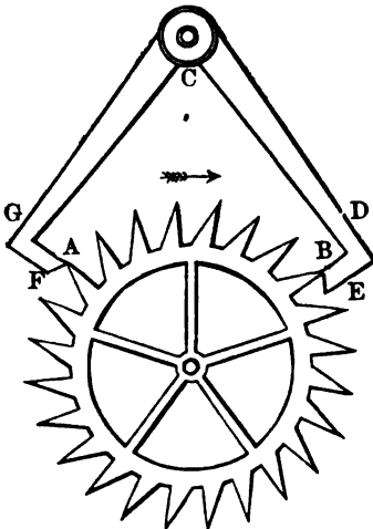
Fig. 5.—Dead Escapement.
