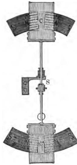
FIG. 17.—Ritchie's Pendulum.
