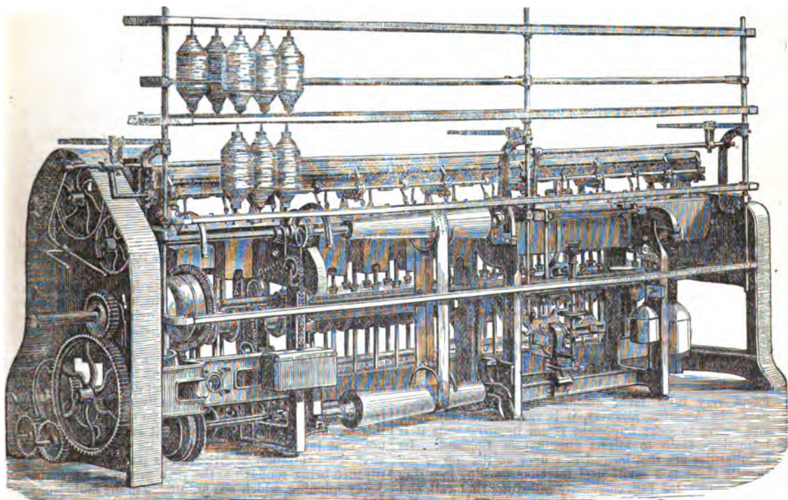
FIG. 10.—Roving Frame.
