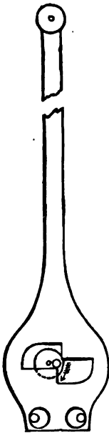
FIG. 7. Maedowall's Escapement.
