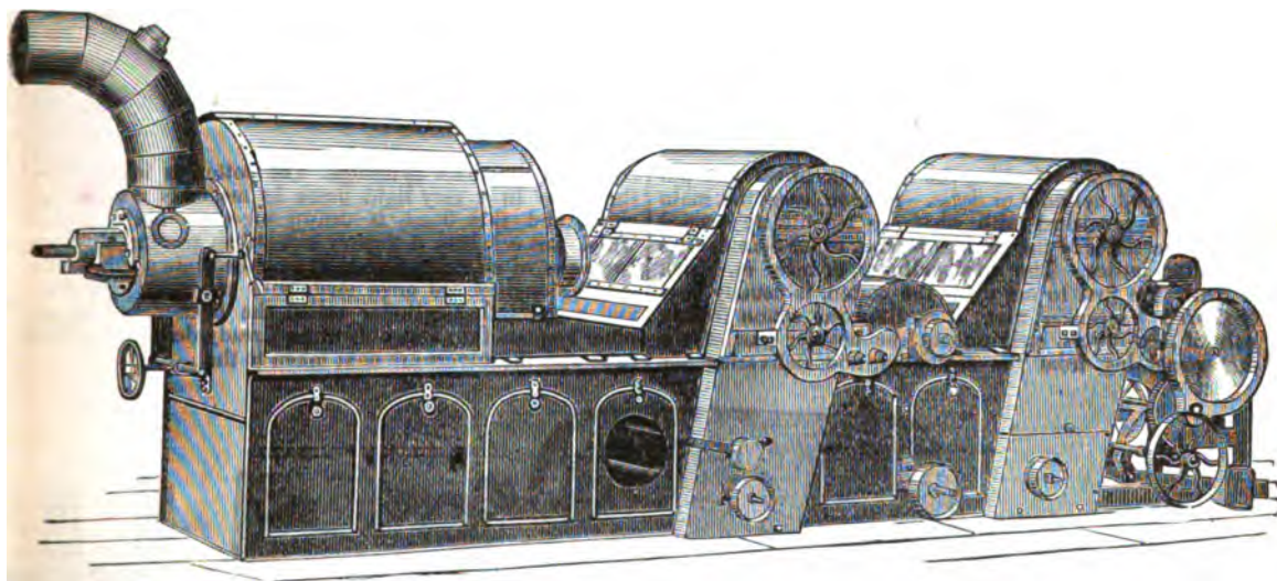
FIG. 2.—Opener.
